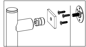
639 RZP ΡΟΖΕΤΑ ΛΑΒΗΣ ΕΞΩΠΟΡΤΑΣ PULL HANDLES ROSETTE
