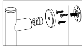
641 RZP ΡΟΖΕΤΑ ΛΑΒΗΣ ΕΞΩΠΟΡΤΑΣ PULL HANDLES ROSETTE
